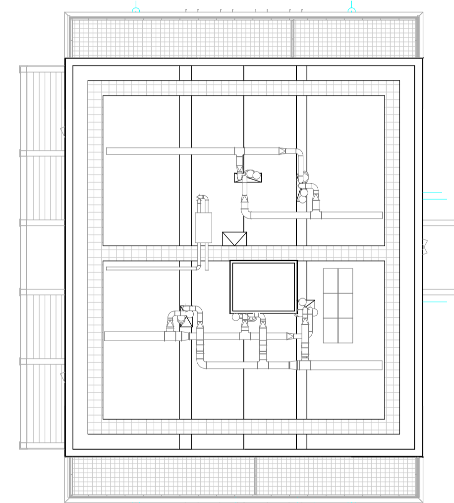
dakaanzicht
