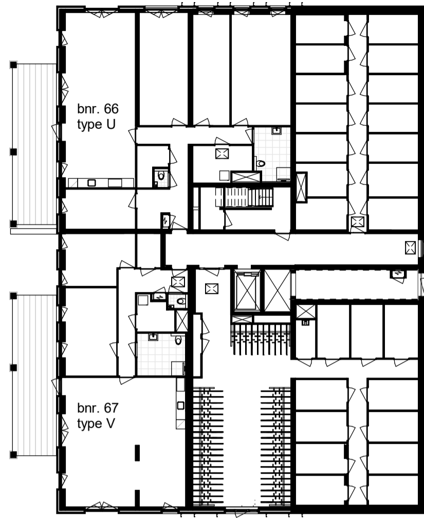
begane grond
