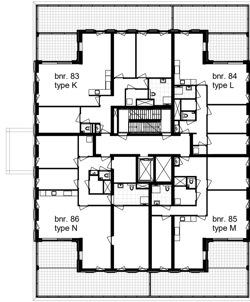
4e verdieping
