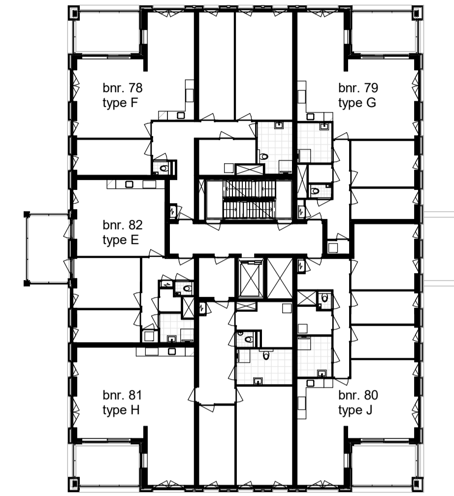
3e verdieping
