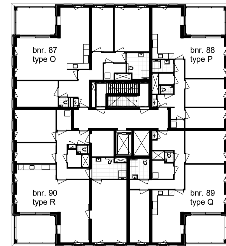
5e verdieping
