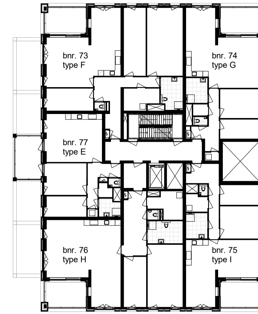
2e verdieping
