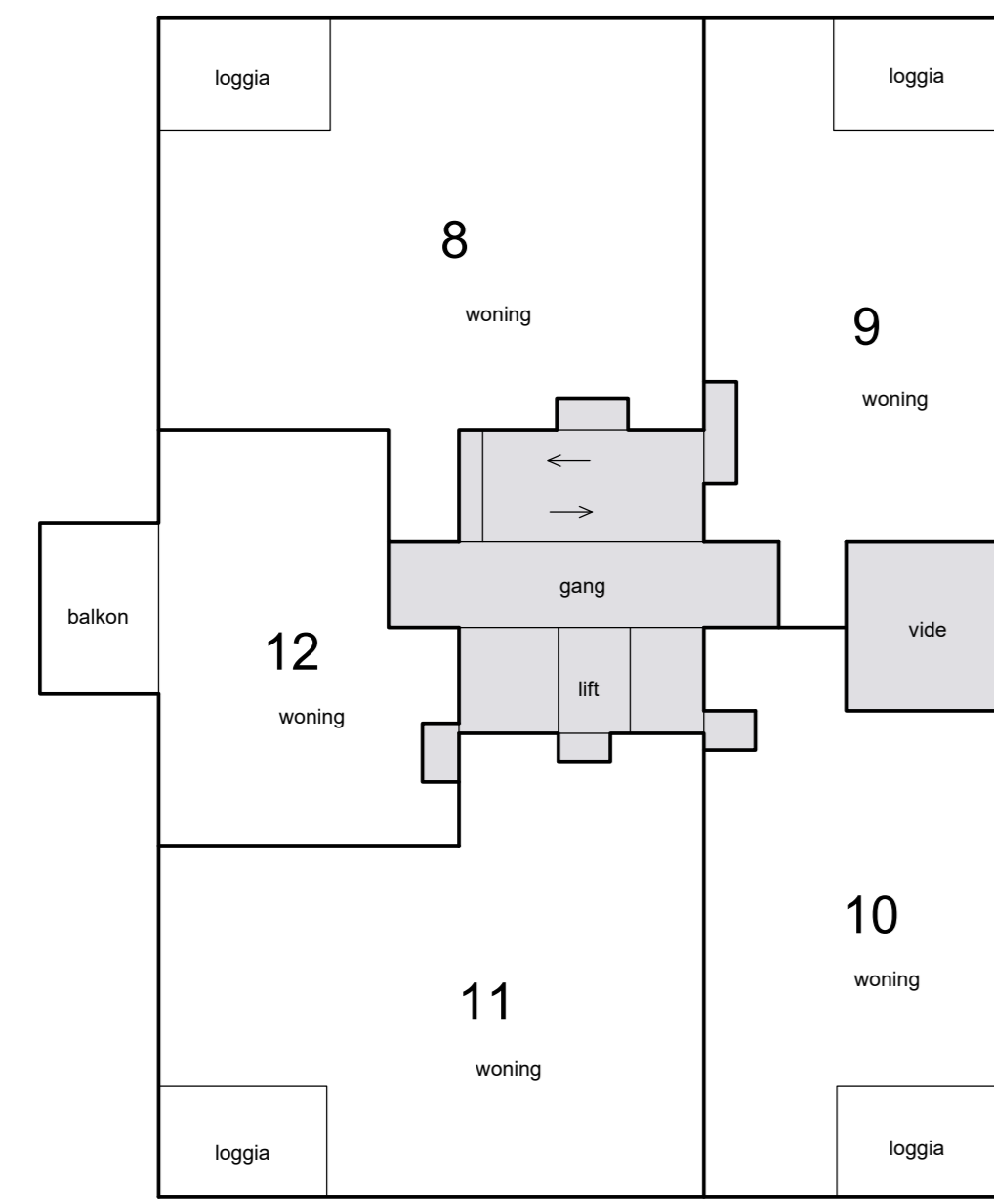
2e verdieping
