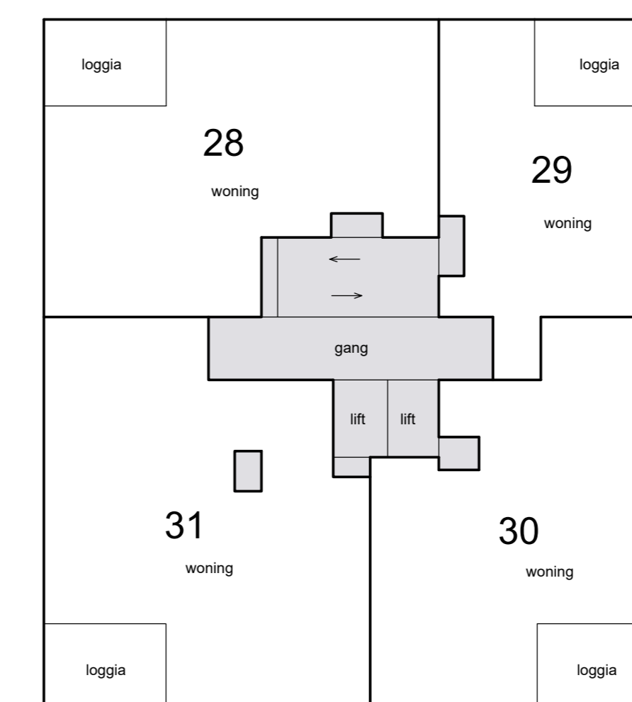
7e verdieping
