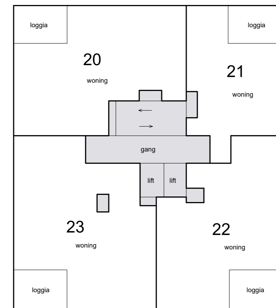
5e verdieping
