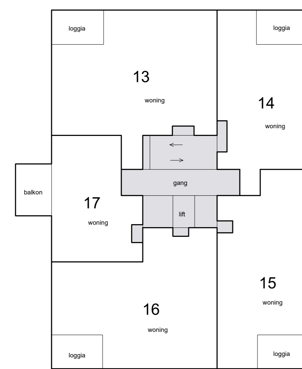
3e verdieping
