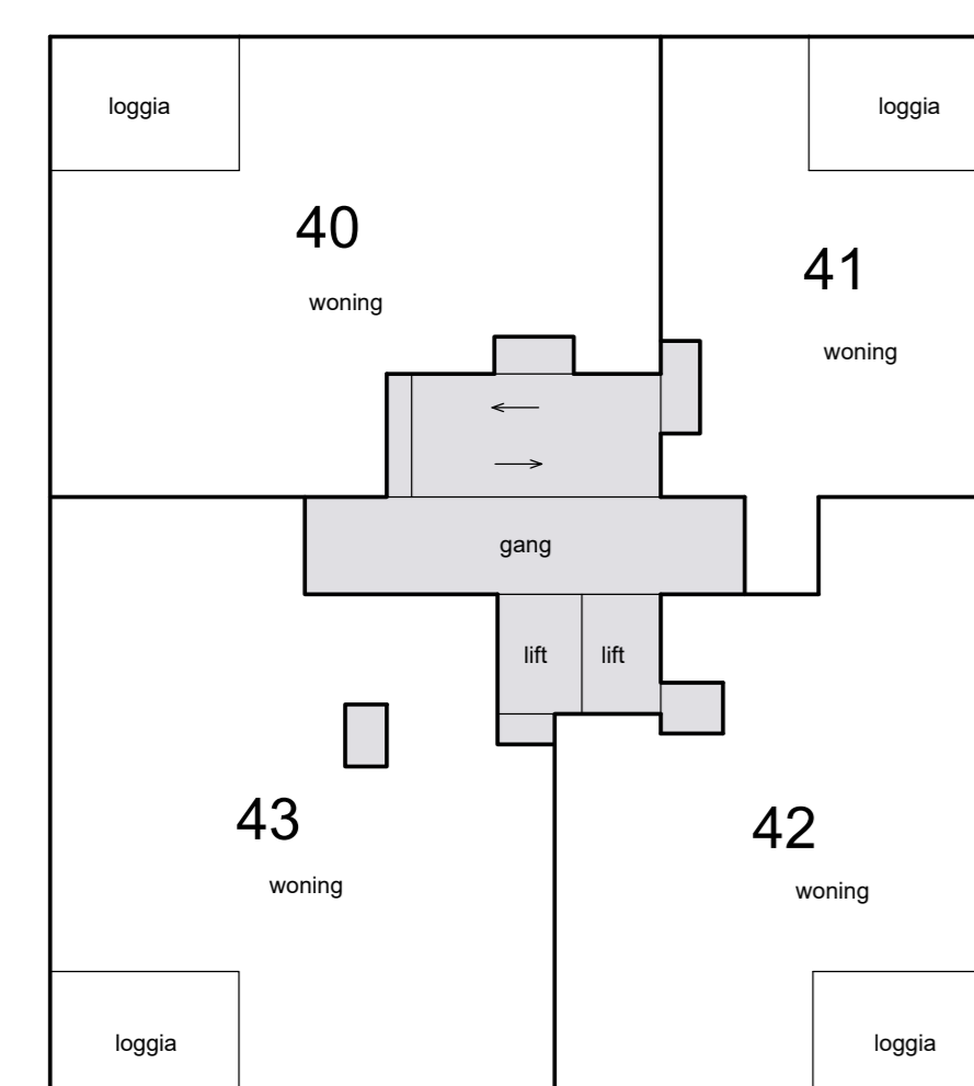
10e verdieping
