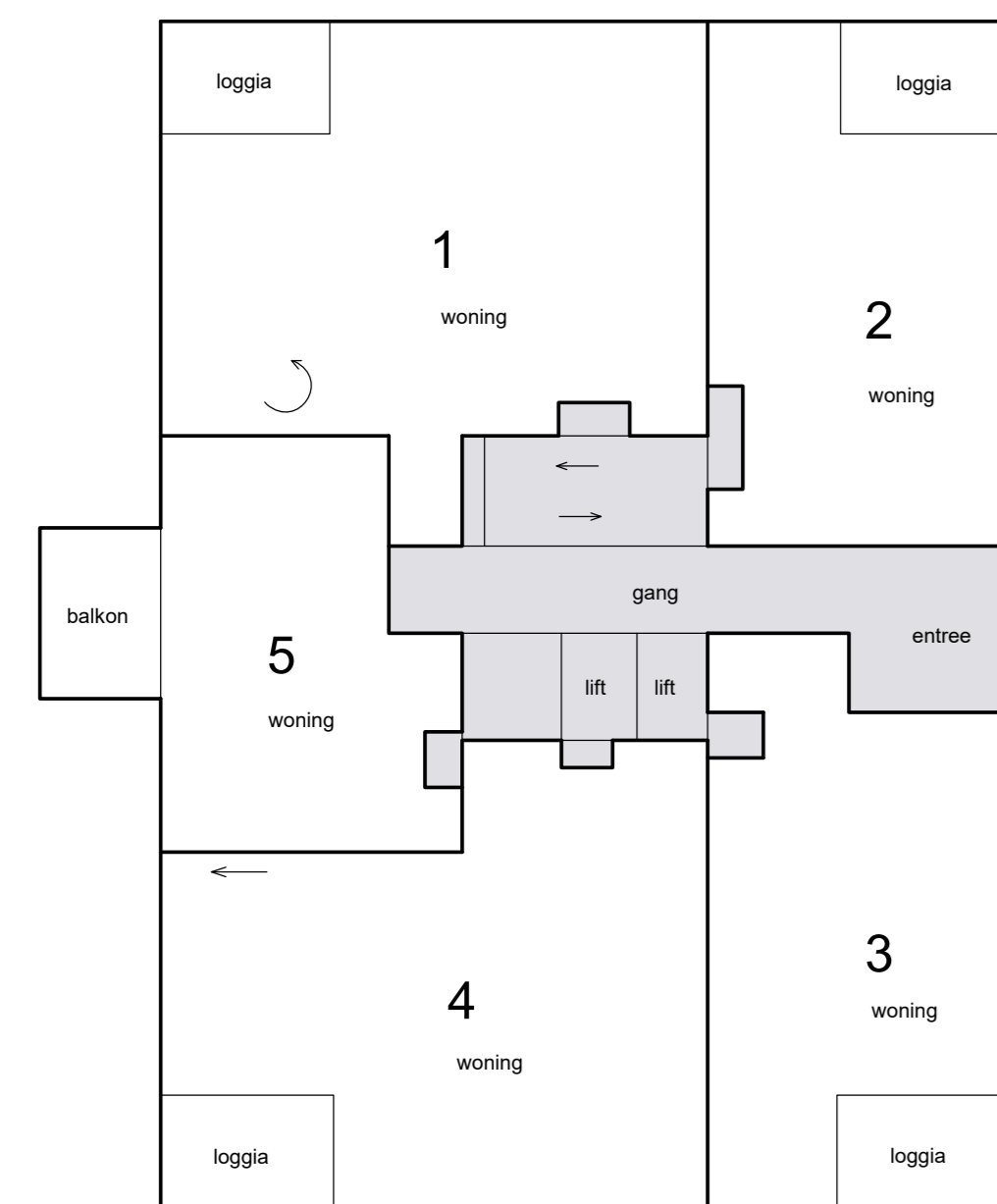
1e verdieping
